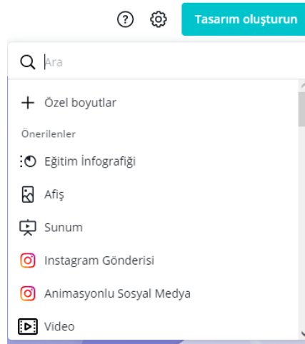
Şekil 4.2 Tasarım oluşturma
