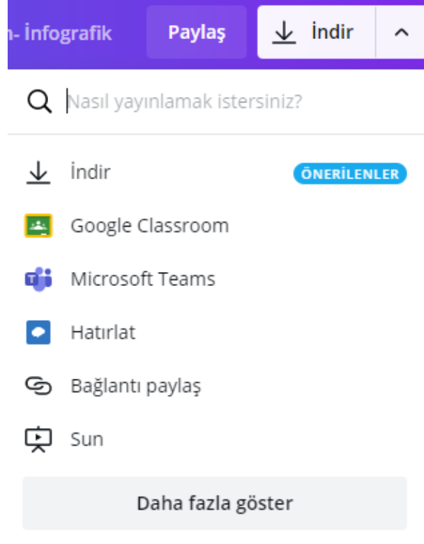
Şekil 5.1 Tasarımın kaydedilmesi
