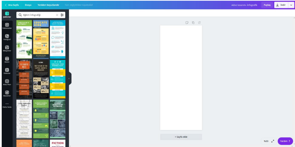
Şekil 4.3 Tasarım oluşturma
