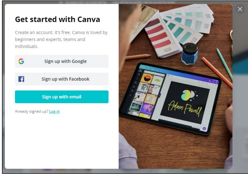
Şekil 3.2 Üyelik sayfası
